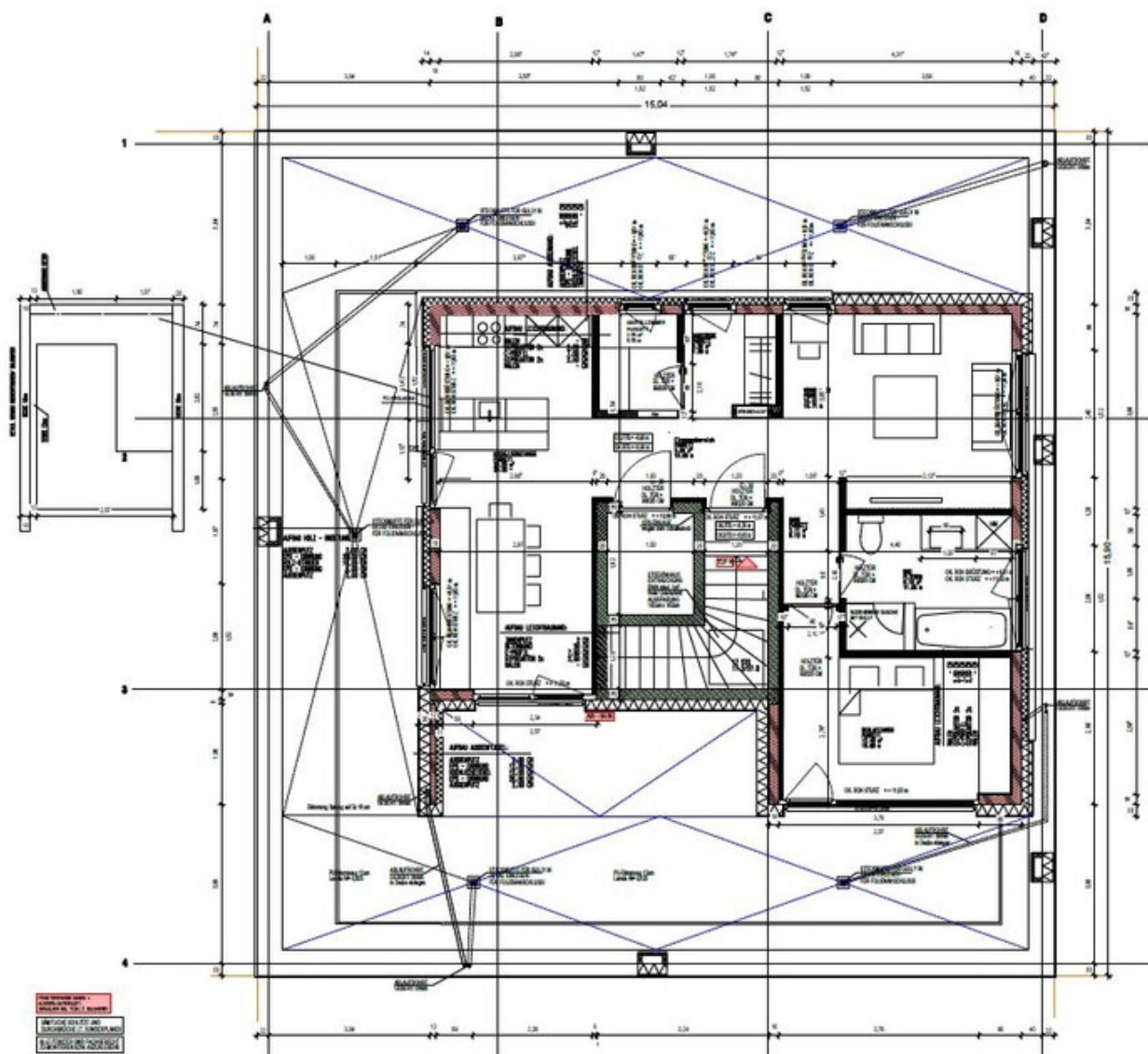
GRUNDRISS DACHGESCHOSS
