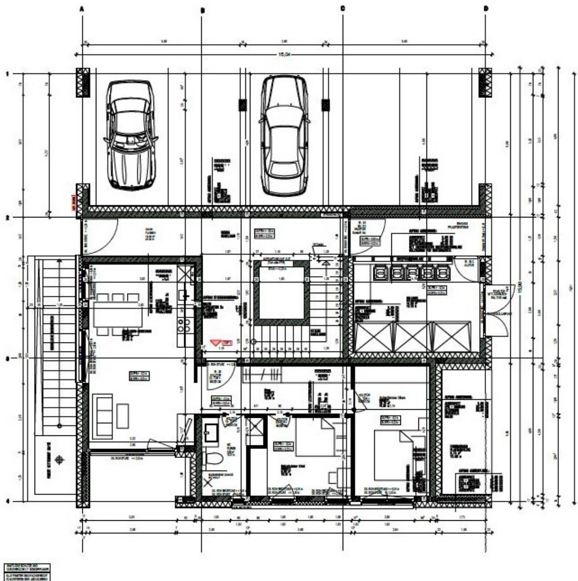
GRUNDRISS ERDGESCHOSS
