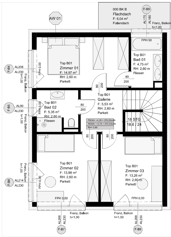
1.OBERGESCHOSS | 1_100
