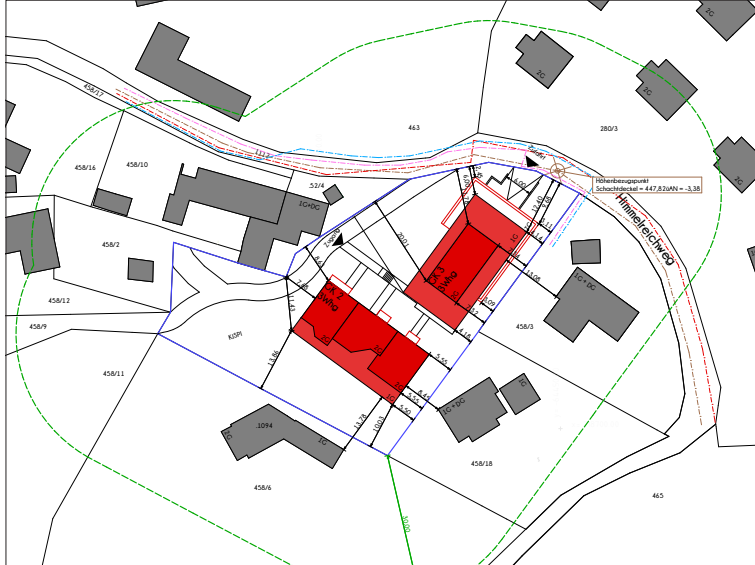
Lageplan
