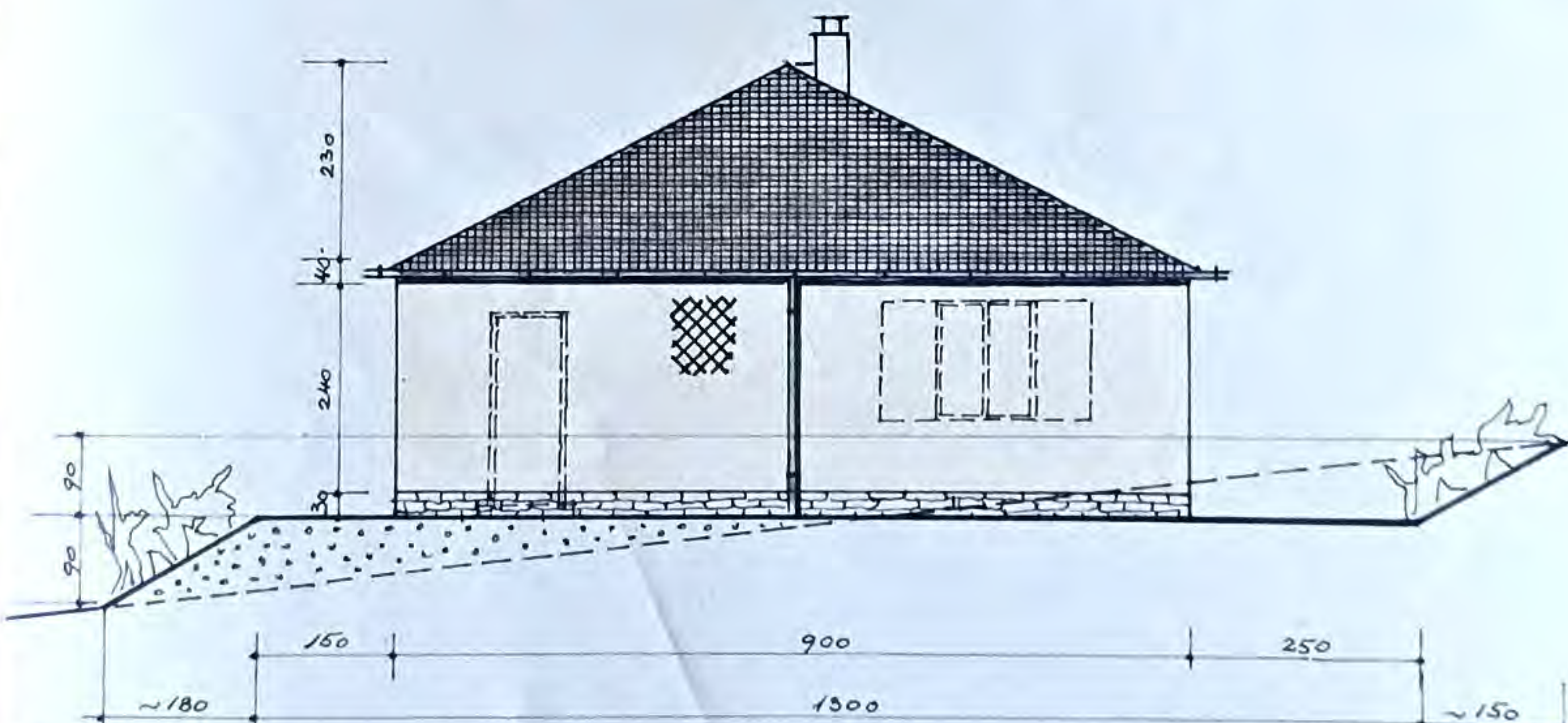
SEITENANSICHT,
