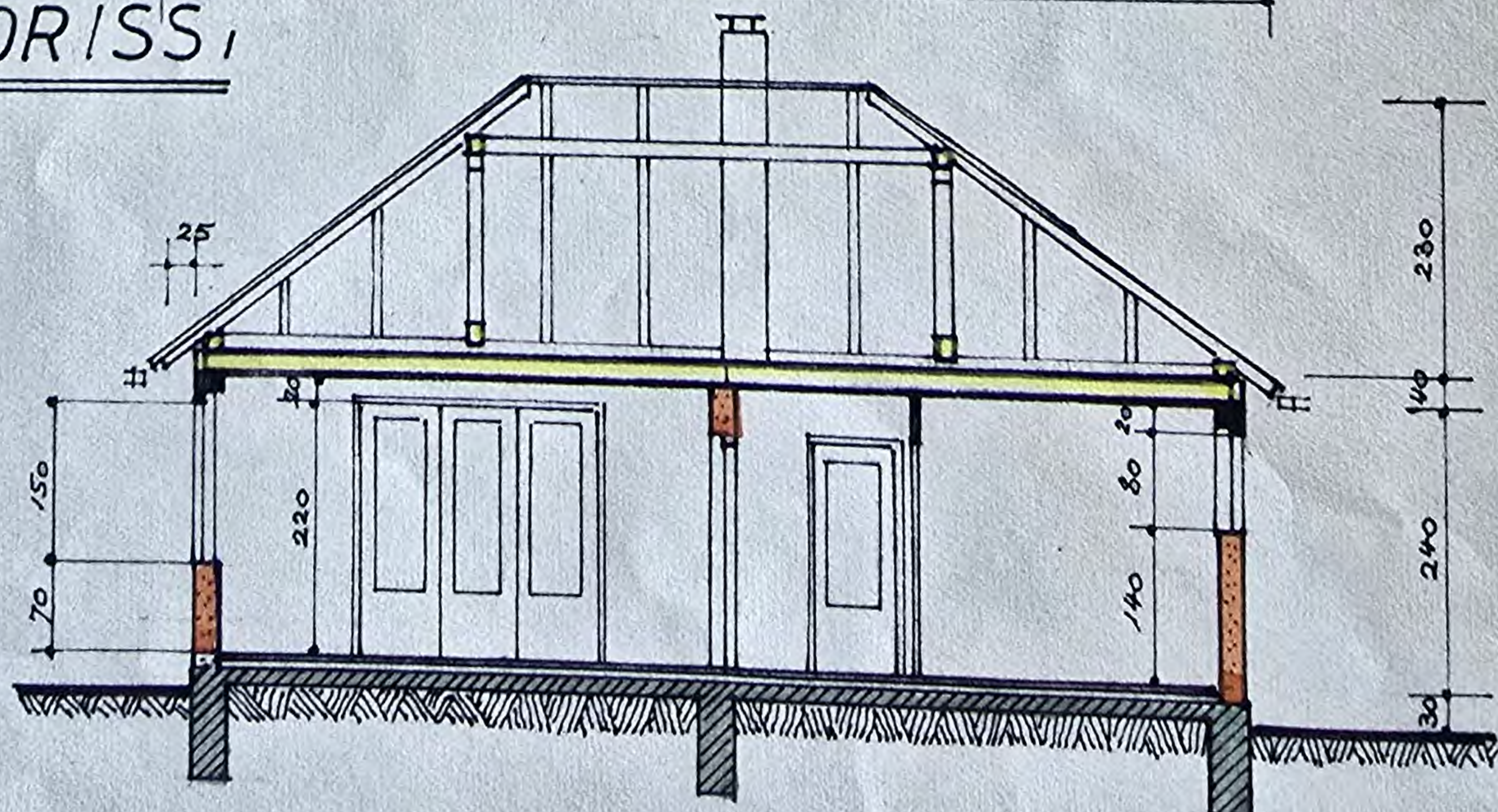
SCHNITT,
