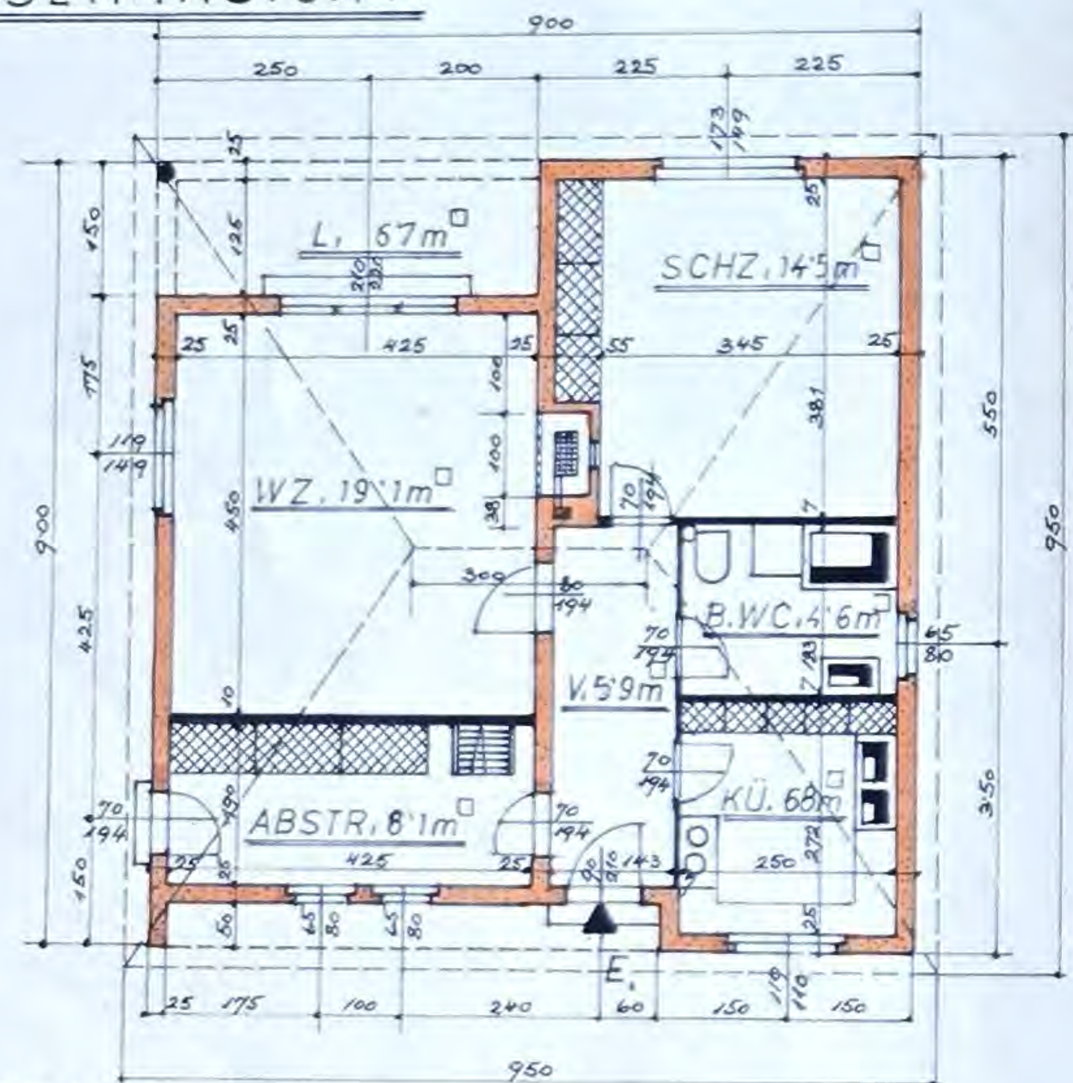
GRUNDRISS,
