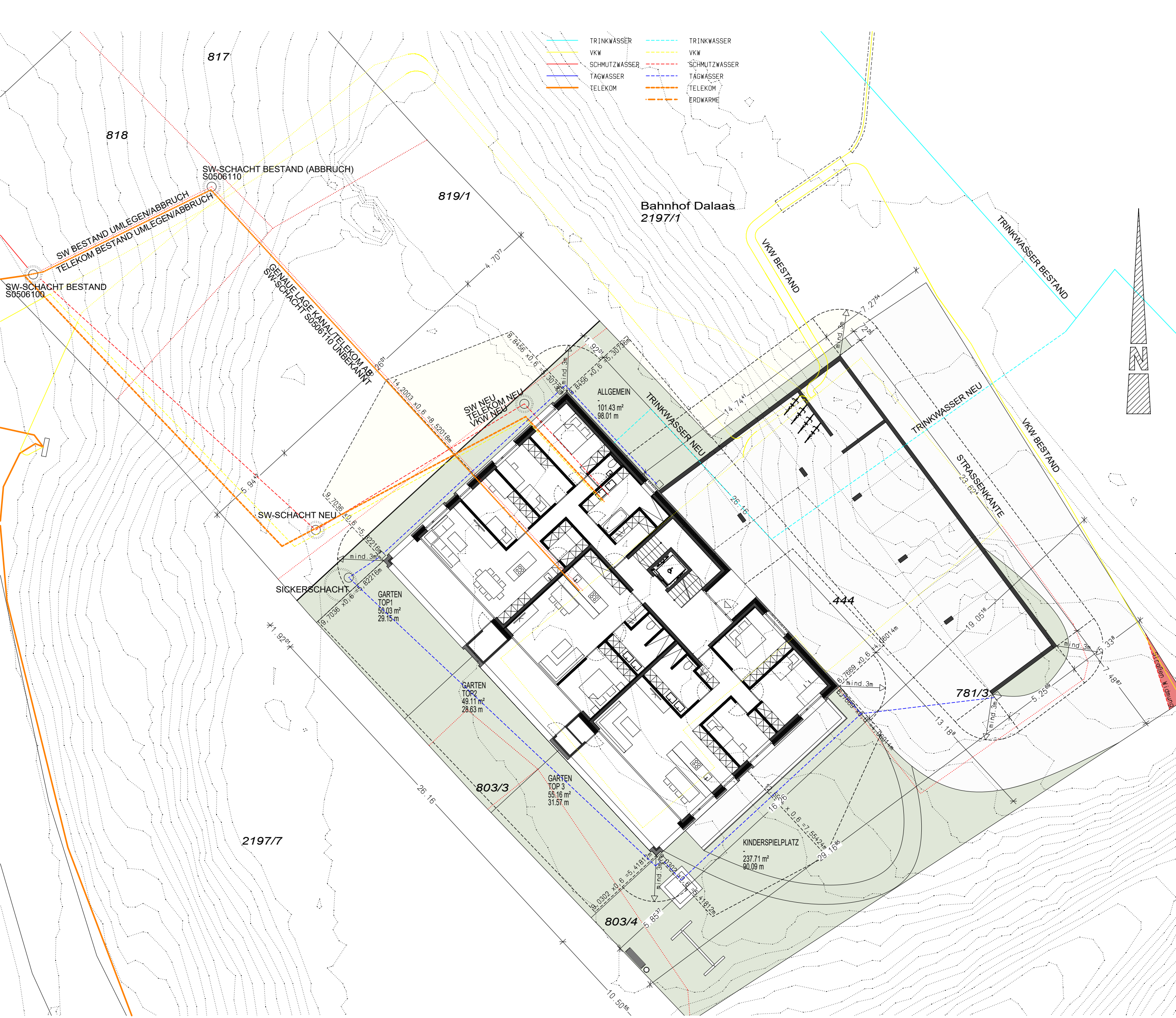
Lageplan M 1:200 inkl. Abstandsflächen
