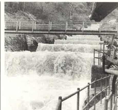
Triebentalbach — Staustufenverbauung.
