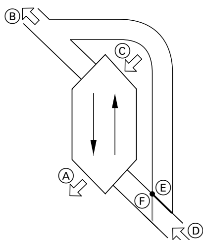
Abb. 69 Beispiel: Vitovent 300-F
