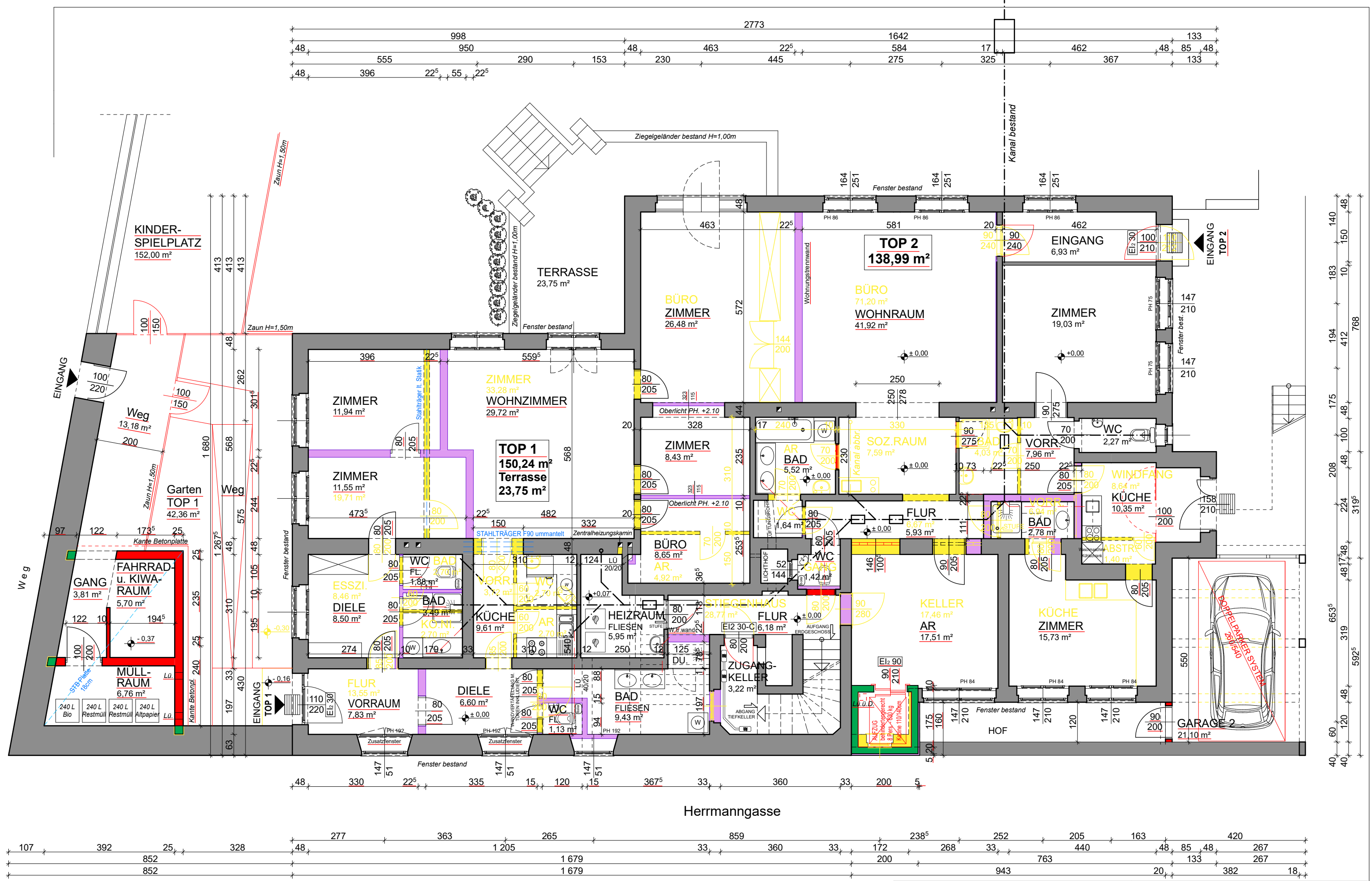
GRUNDRISS UNTERGESCHOSS M 1:100
