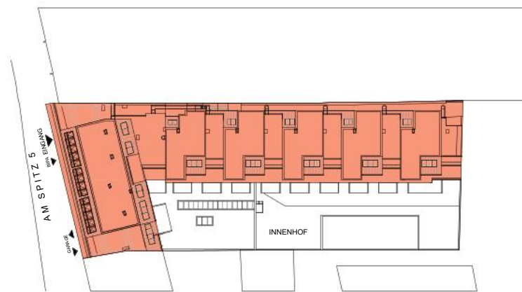
LAGEPLAN M 1:1000
