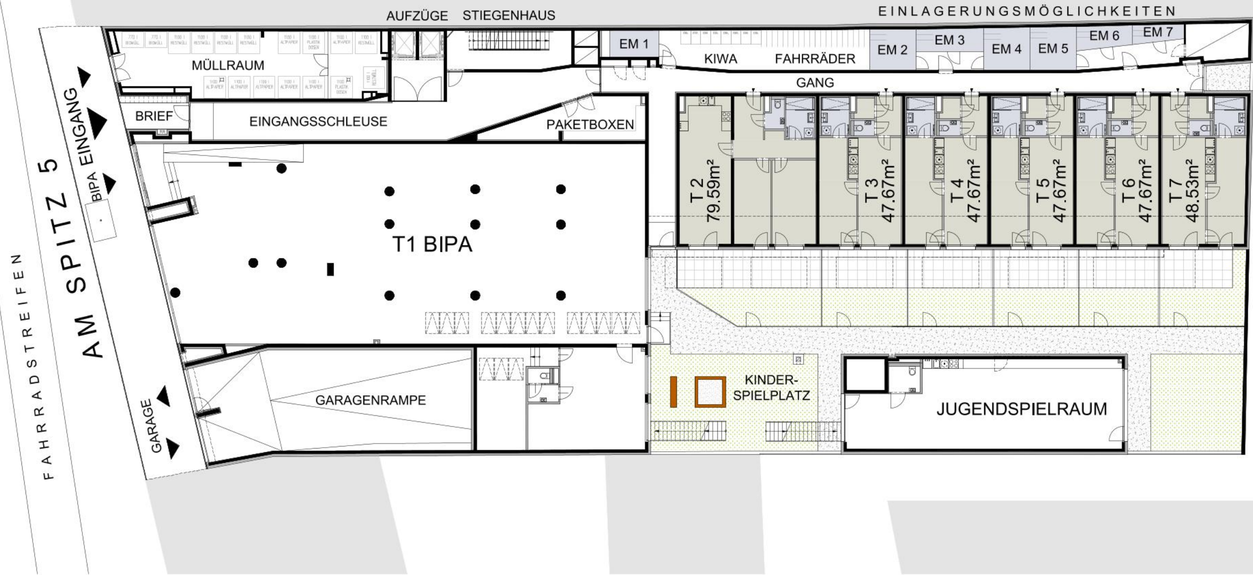
ERDGESCHOSS
