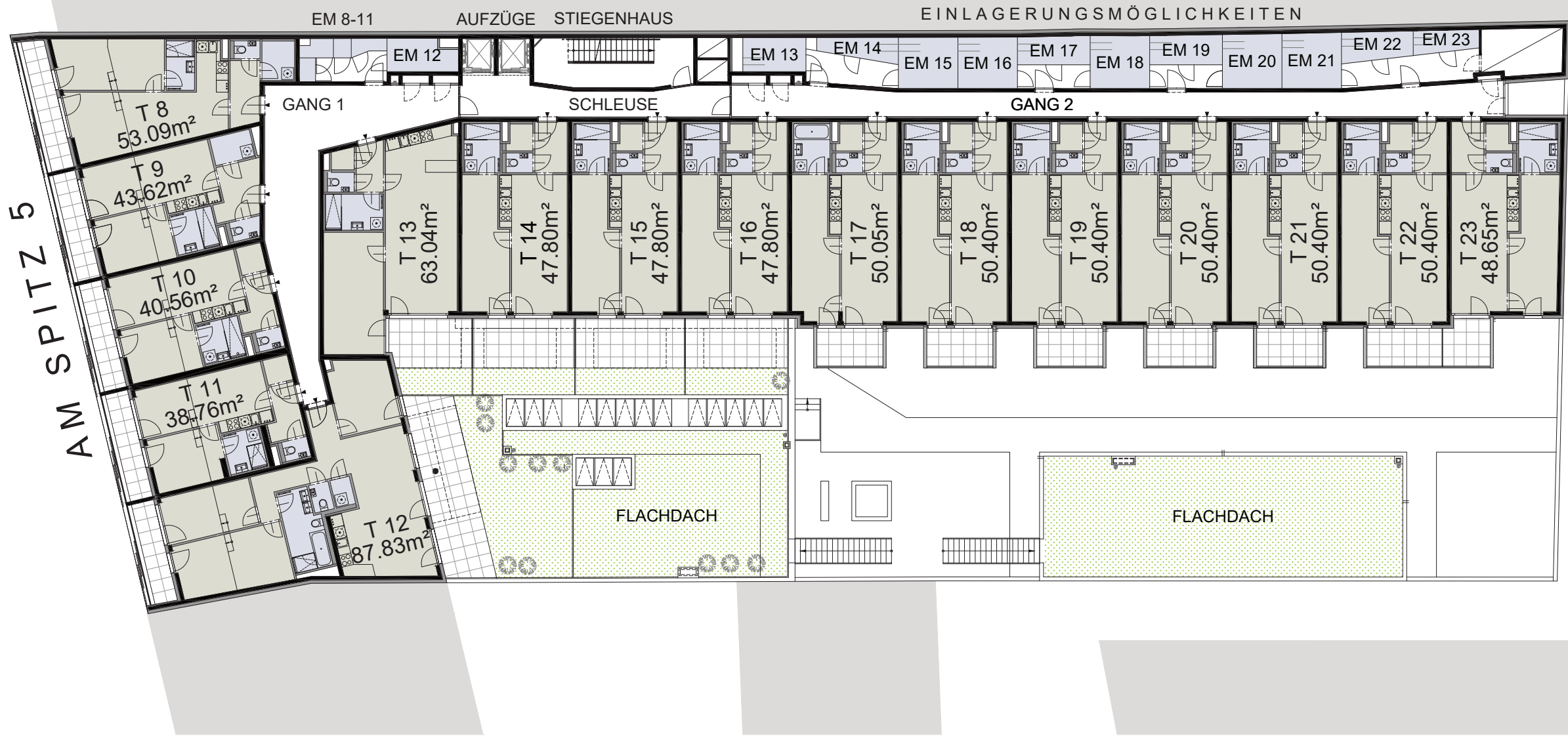
1. OBERGESCHOSS
