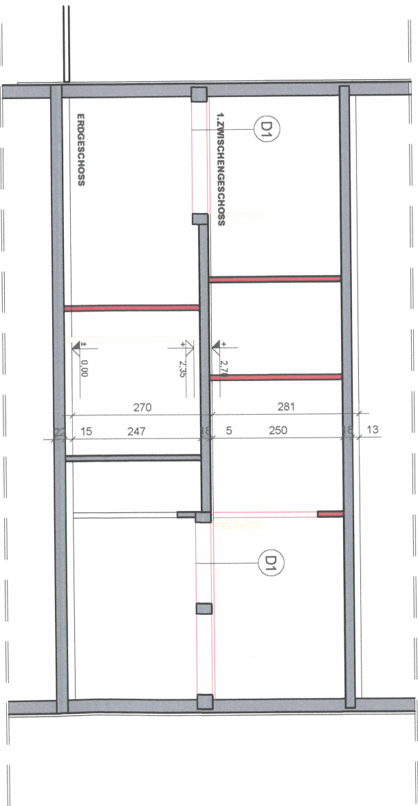
SCNITT A-A
