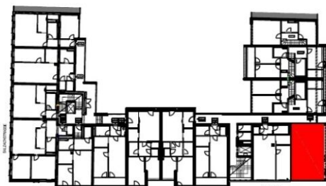
LAGEPLAN 3.OBERGESCHOSS
