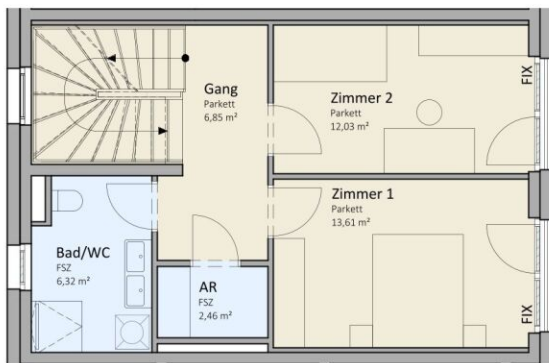
1. Obergeschoß
