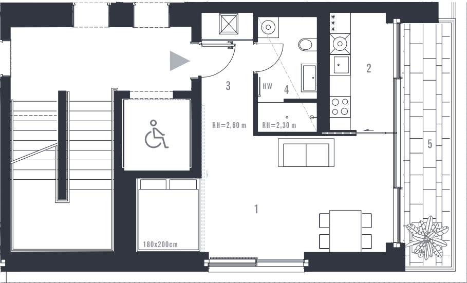
Obergeschoss top floor
