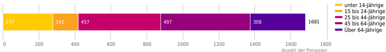
Altersverteilung (Wundschuh)
