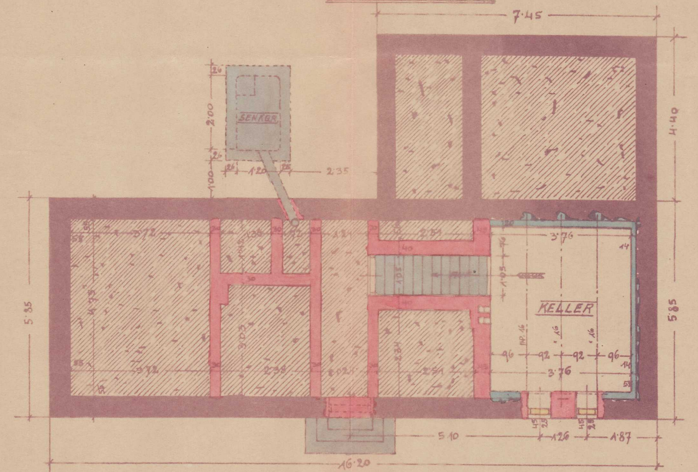
KELLERGEßCHOSS
