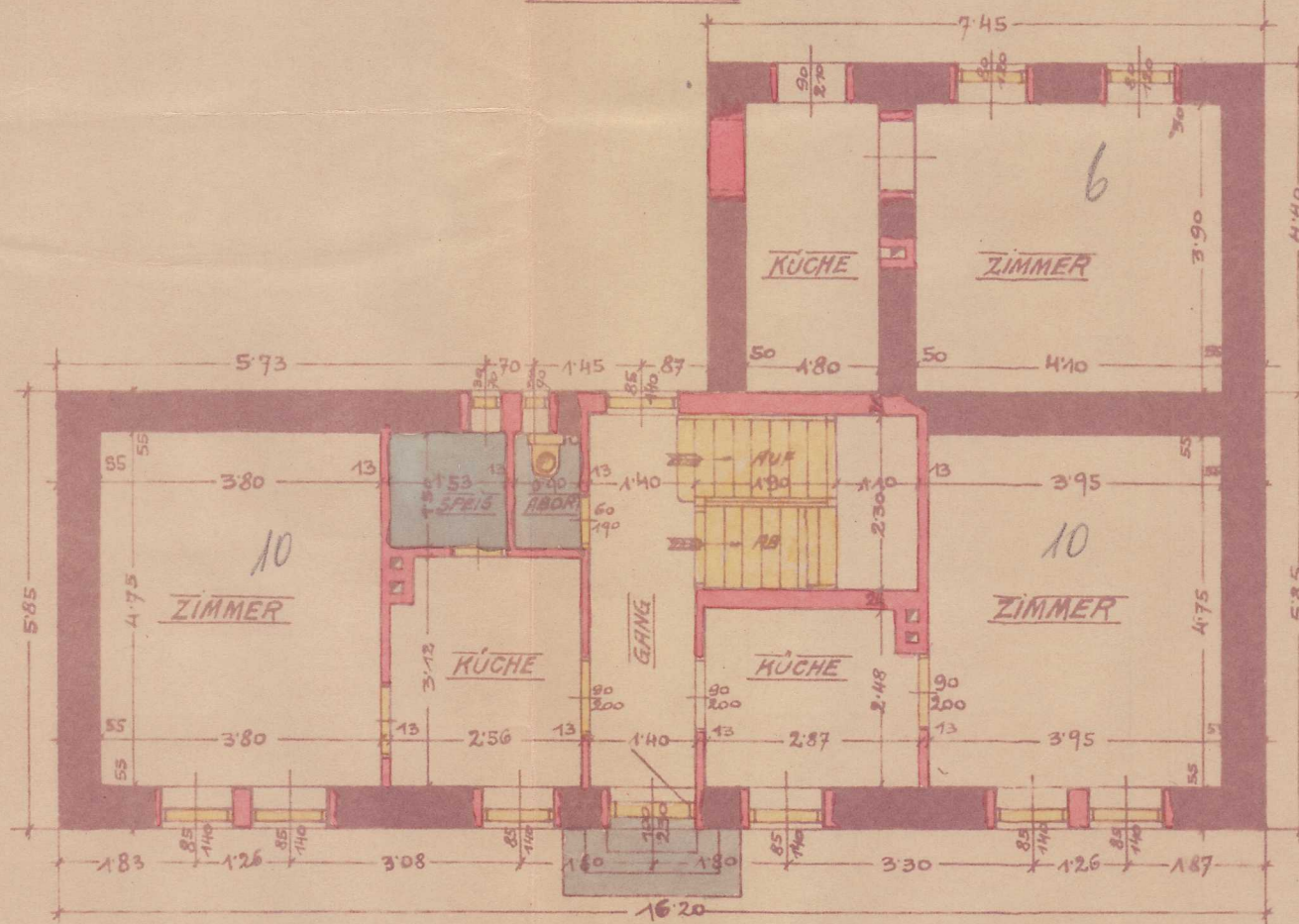
PARTERRE
