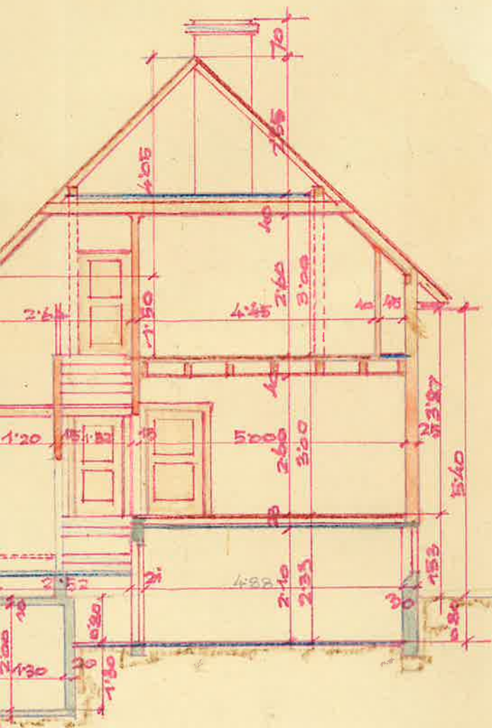
Querschnitt: ab
