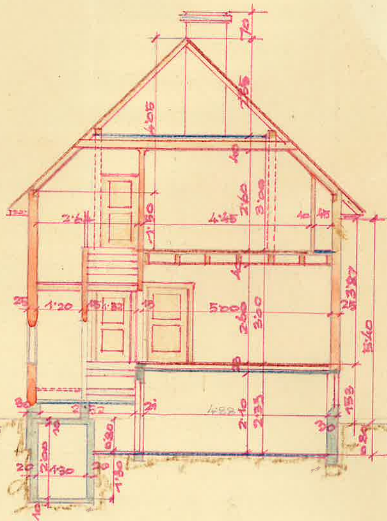
Querschnitt ab
