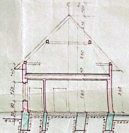
Schnitt A-B
