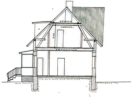
SCHNITT.
