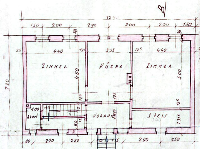
Porterre - Grundriss.
