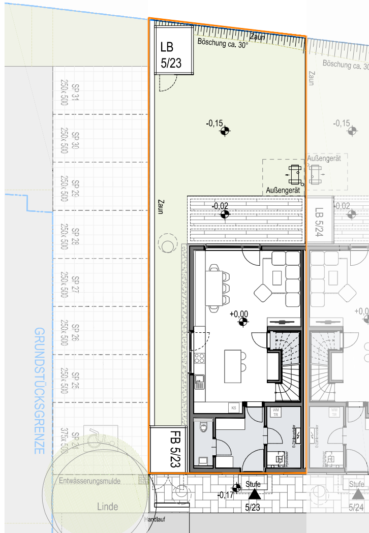
ERDGESCHOSS
