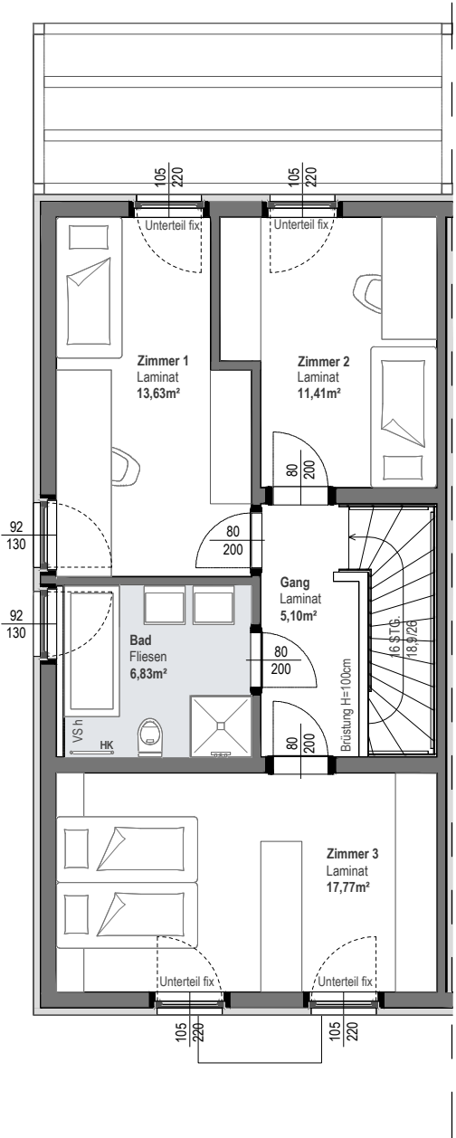
OBERGESCHOSS
